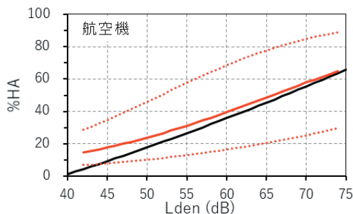
図-2 航空機騒音に対する曝露-反応関係の比較
